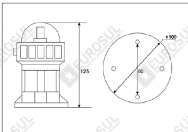
1. Dimensões
